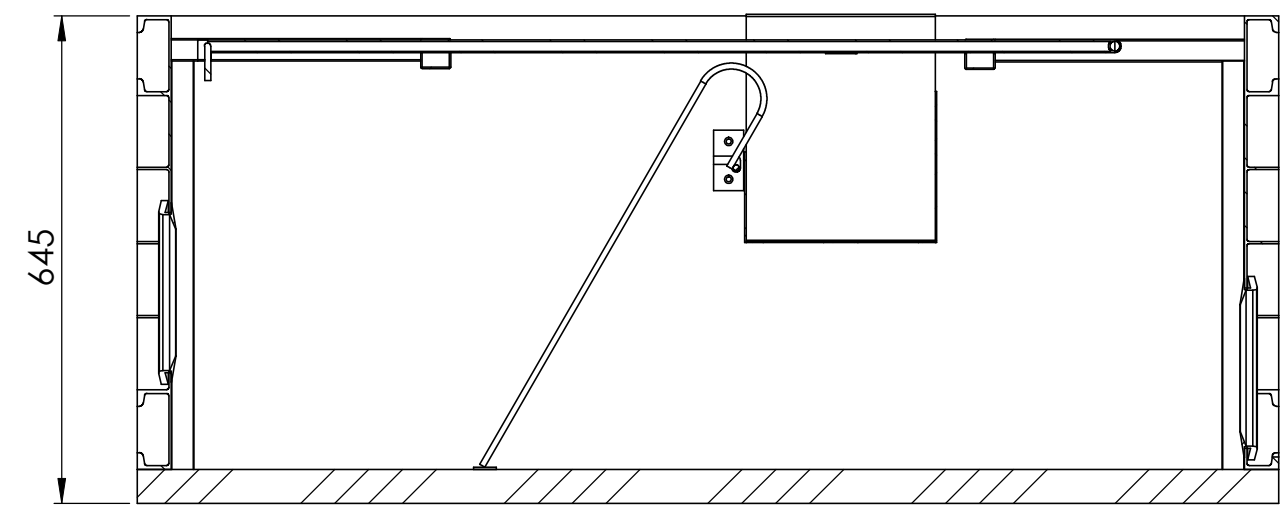
COUPE A-A
