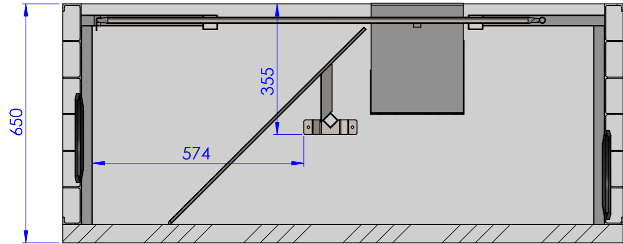
COUPE A-A
